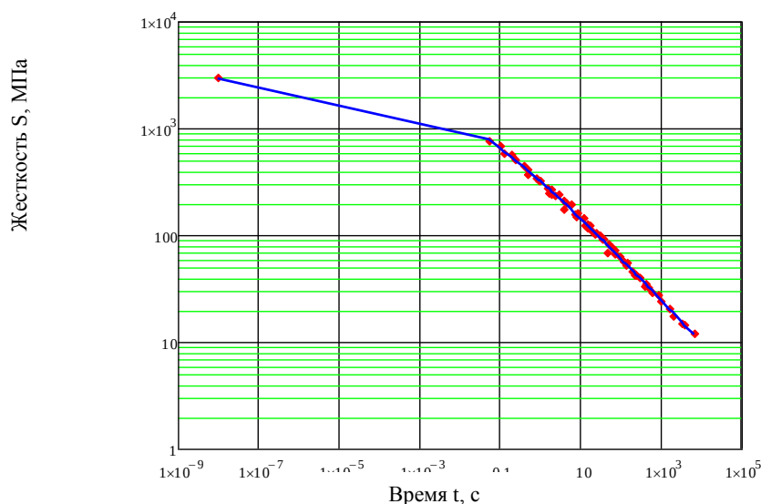
Рисунок 6. Сглаживание обобщенной кривой жесткости битума при температуре -22,2 °С.
