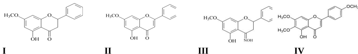
Рисунок 1 – Химические формулы изучаемых флавоноидных соединений: Пиностобин (I), Тектохризин (II), Оксипиностробина III и Сальвегинин IV.
