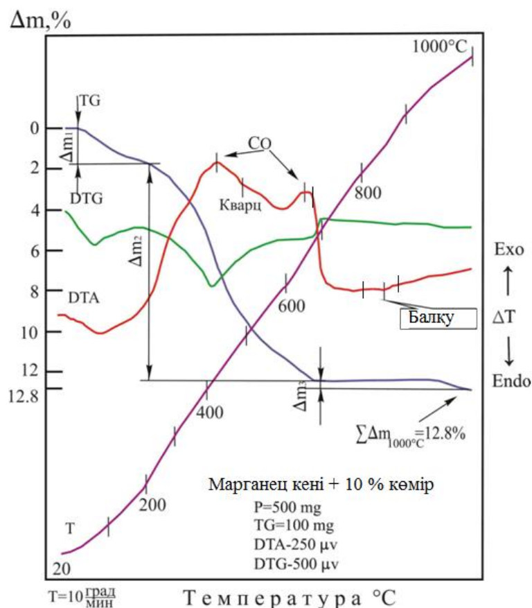
2 – сурет. «Қармола» марганецқұрамдас кеннің көмір қосып түсірілген дериватограммасы
