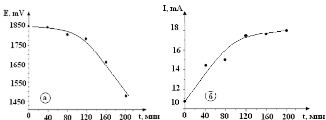
2-сурет. Амальгамаланған алюминий-графит гальваникалық жұбындағы электродтар арасындағы электр қозғаушы күш (а) пен қысқа тұйықталған ток (б) мөлшерлерінің уақыт бойынша өзгеруі: NaCl-100г/л, K_3[Fe(CN)_6] -10 г/л және K_4[Fe(CN)_6] -10 г/л.
