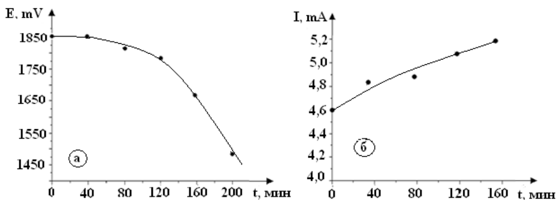
3-сурет. Амальгамаланбаған алюминий-графит гальваникалық жұбындағы электродтар арасындағы электр қозғаушы күш (а) пен қысқа тұйықталған ток (б) мәндерінің уақыт бойынша өзгеруі: NaCl-100г/л, K_3[Fe(CN)_6] -10 г/л және K_4[Fe(CN)_6] -10 г/л.
