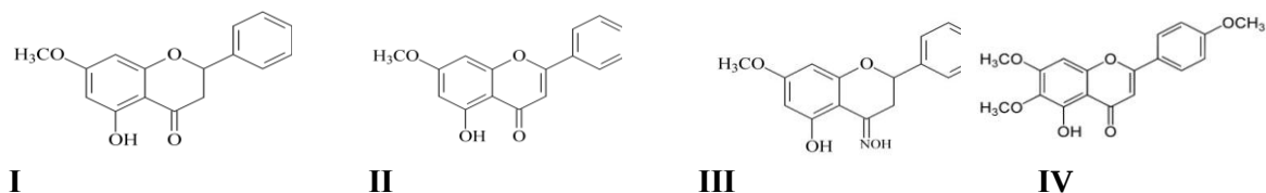
Рисунок 1 – Химические формулы изучаемых флавоноидных соединений: Пиностин (I), Тектохризин (II), Оксипиностробин III и Сальвегинин IV.
