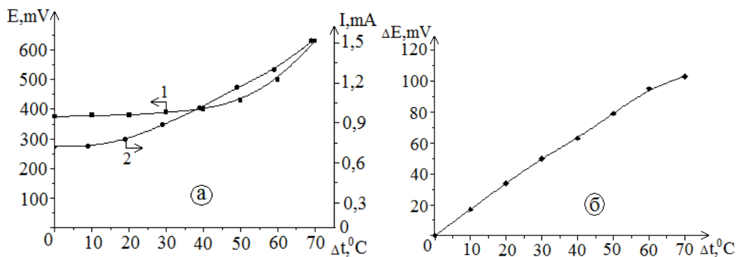
Рисунок 1 – а) Зависимость изменения величины ЭДС(1) и ТКЗ(2) между свинцовым и графитовым электродами от разности температуры; б) – влияние изменения температуры раствора на изменение ред-ок потенциала графитового электрода.
