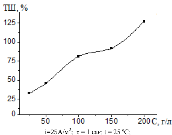
2-сурет – Композициялы күкірт электродының анодты поляризацияланғанда сульфат иондарының түзілуінің тотығуының ток бойынша шығымына NaCl концентрациясының әсері
