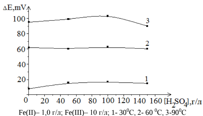
Рисунок 7 - Изменение величины ред-окс потенциала графитового электрода от концентраций серной кислоты при различных температурах термостатированного пространства электролизера
