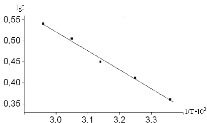
7 – сурет – Калий иодиді ерітіндісінде \lg I мәнінің температураға ( 1/T \cdot 10^3 ) тәуелділігі ( \Delta E=0,55\text{B} )
