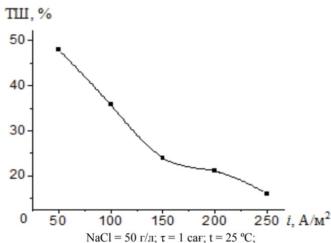
1-сурет – Анодты поляризацияланған композициялы күкірт-графит электродындағы ток тығыздығының сульфат иондарының түзілуінің ток бойынша шығымына әсері
