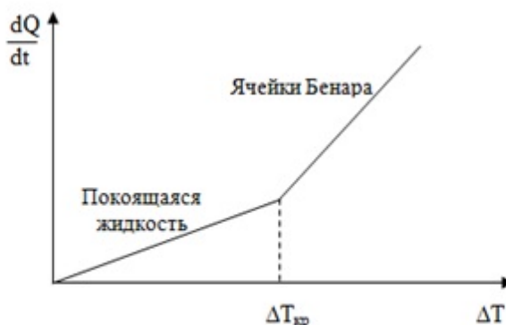
Рисунок 25. Зависимость скорости переноса теплоты от разности температур
