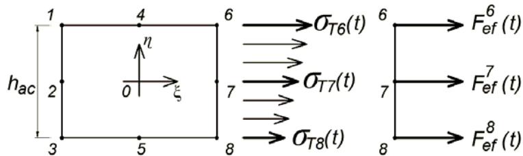
Рисунок 7. К определению эффективных узловых сил
