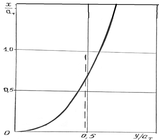
Рисунок 1 – Глубина проникновения и траектория факела ГТ-6 и ПГСПГ ТТЭЦ-2
