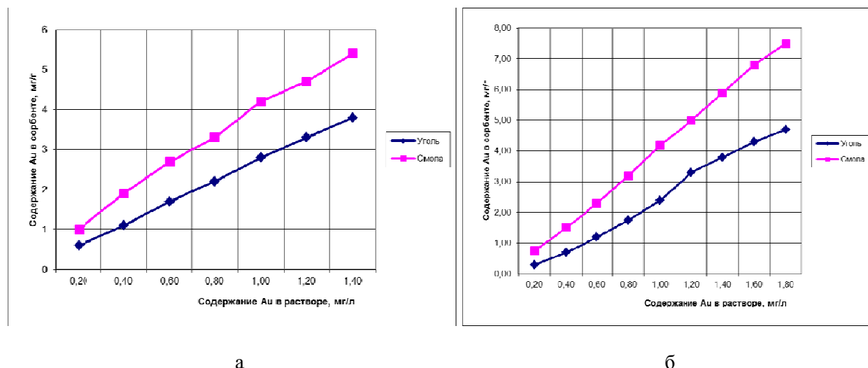
а б Выщелачивающий раствор приготовлен при растворении NaCN в алматинской водопроводной воде (а) и оборотной воде действующего рудника (б)
