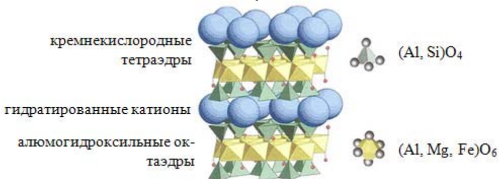
Рисунок 1 - Строение монтмориллонита
